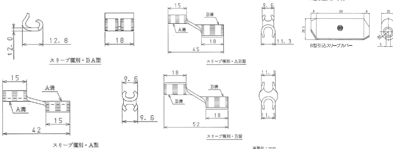
付図 低圧引込スリーブ
