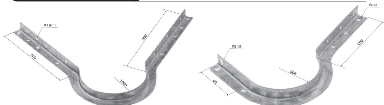
R形アーム：関西電力型 MRA-KD
