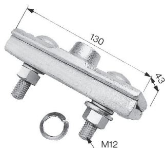
SS 用吊架金物 (タルミ付) [KTSS]
