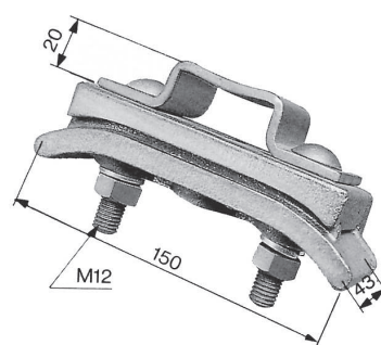
SS 用曲り吊架線金物 [KTSM]
