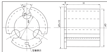
東京電力型 分岐バンド用ゴムスペーサー
