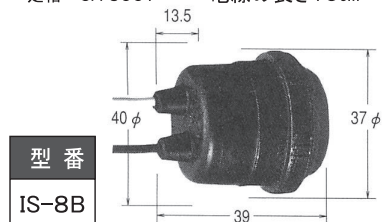
外形寸法—37φ
