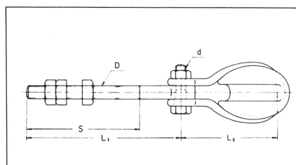
W \frac{1}{2} フックボルト+玉碍子
