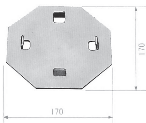
沈下防止板 UCI
