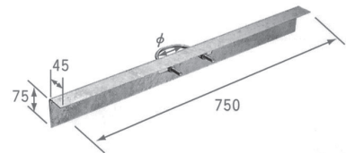
ボール根枷 Uボルト付 φ 90-Z UPN-90 φ 115-Z UPN-115 φ 140-Z UPN-140
