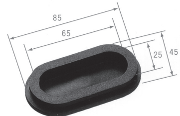
ゴムブッシングD UGBD
