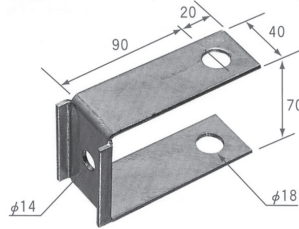
引留金物 UHK
